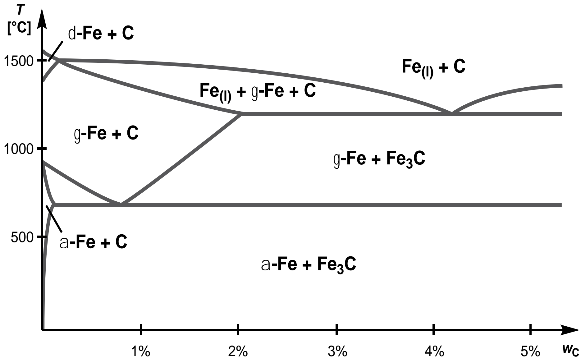
Abb. 1.1: Vereinfachtes Phasendiagramm des Eisen-Kohlenstoff-Systems in Abhängigkeit vom Massenanteil an Kohlenstoff. \text{Fe}_3\text{C} beschreibt die metastabile Verbindung Zementit. (Nicht beschriftete Bereiche können vernachlässigt werden.)
