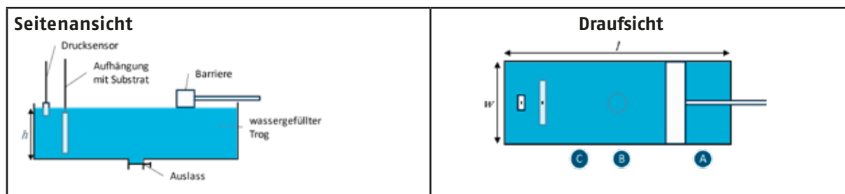
Abbildung 4: Versuchsaufbau zur Übertragung von Tensid-Monolagen auf ein Substrat
