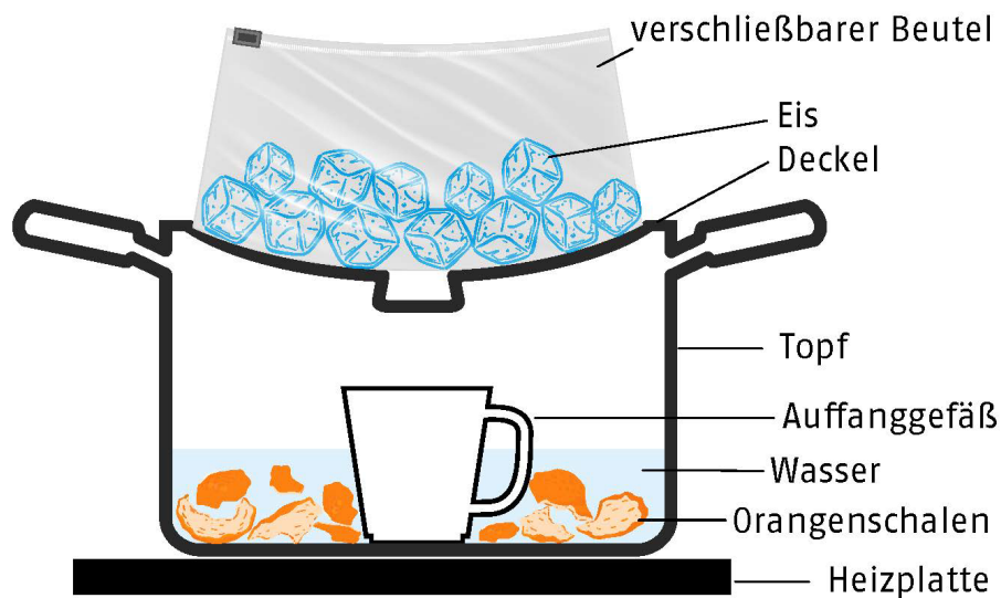
Abbildung 1: Versuchsaufbau
