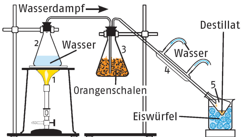
Abbildung 2: Labor-Apparatur
