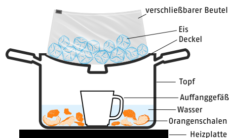
Abbildung 1: Versuchsaufbau
