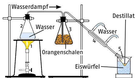
Abbildung 2: Labor-Apparatur
